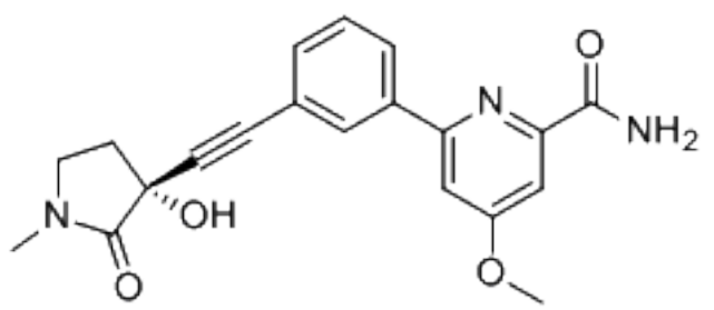
PC-6251401, DMSO-d6
